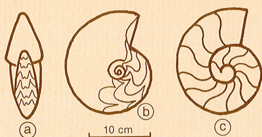
3. GONIATITE
