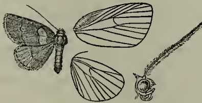
Dastira hippialis , ♂. \frac{3}{2} .
