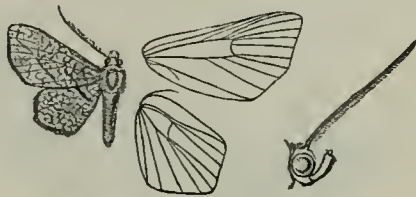
Macrogonia igniaria , ♂ \frac{1}{2} .
