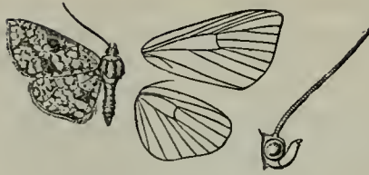
Plagiosella clathrata , ♂. \frac{3}{2} .
