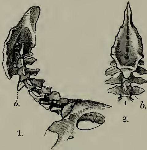
Toccus erythrorhynchus . Caudal vertebræ. 1, lateral view; 2, ventral view. P, pelvis; b, free intercentrum.
